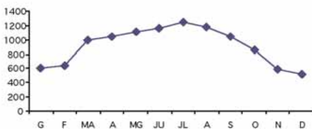
Previsió de la producció d'energia elèctrica al llarg d'un any (Kw-h)
